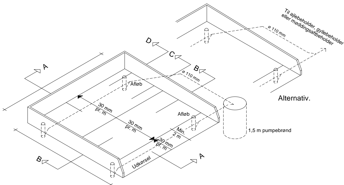
Figur 1.9 Eksempel på korrekt konstruktion af møddingsplads med afgrænsningsmur og fald mod afløb. Kilde: Landbrugets Byggeblade, Arkiv nr. 103.06-05
